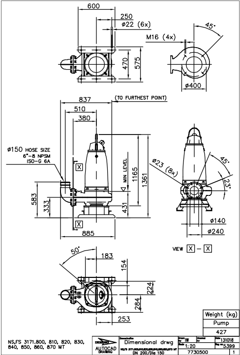
Рис. 32: Установка MT, S
