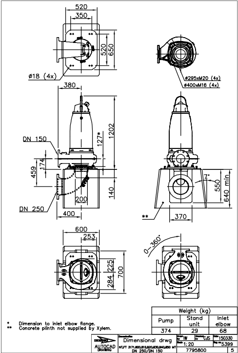
Рис. 34: Установка MT, T
