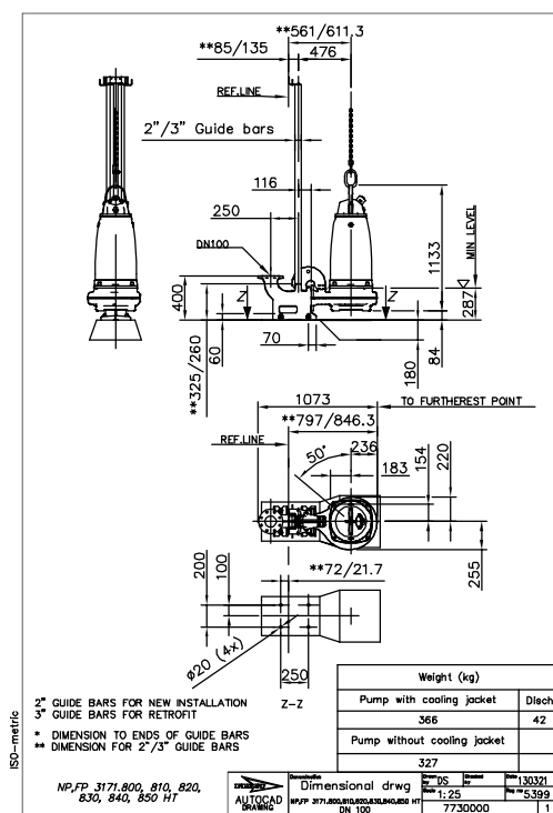
Рис. 37: Установка HT, P
