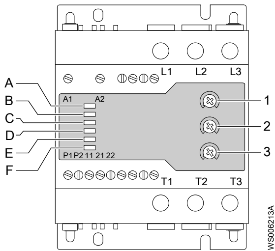
Рис. 8: Разводка клемм устройства плавного пуска
