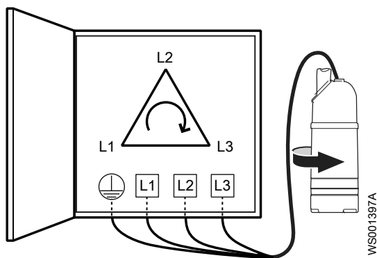
Рис. 4: Включите насос
