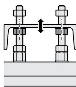
Рис. 61: Регулировка по вертикали
