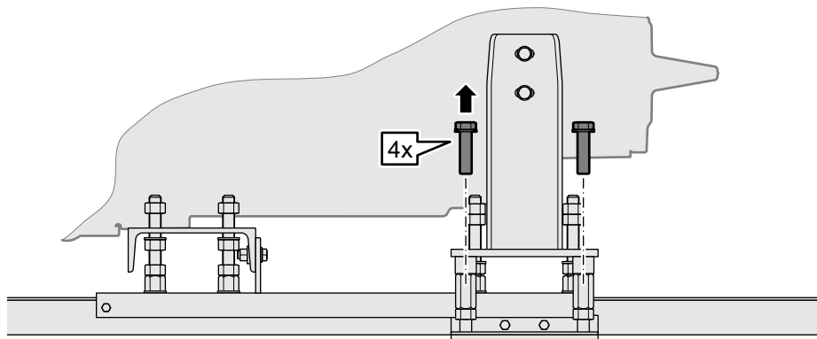
Рис. 52: Снятие болтов
