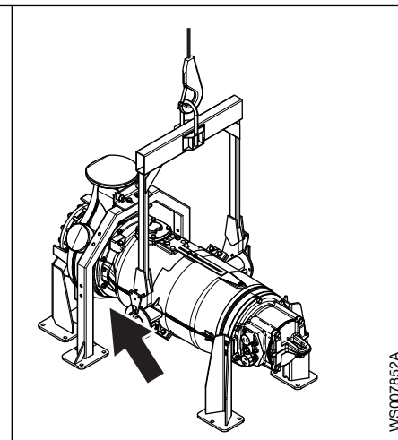
Рис. 50: Отсоединение привода от гидравлического блока
