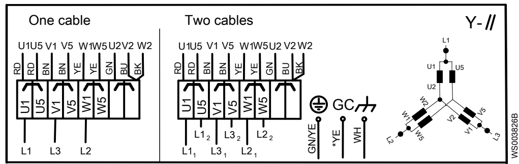
Рис. 12: параллельное соединение «звезда»
