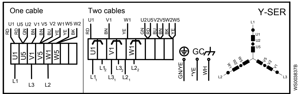
Рис. 13: последовательное соединение «звезда»
