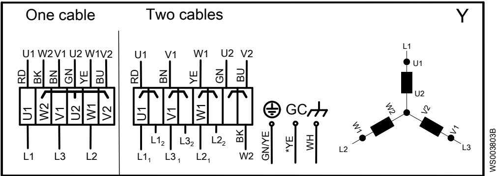
Рис. 8: Соединение “звездой”
