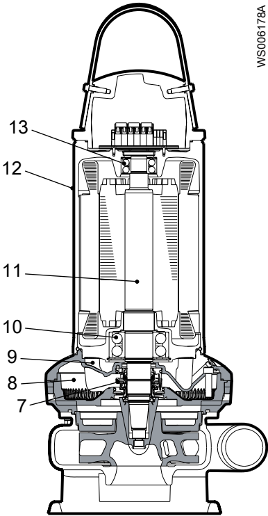
Рис. 1: Без рубашки охлаждения
