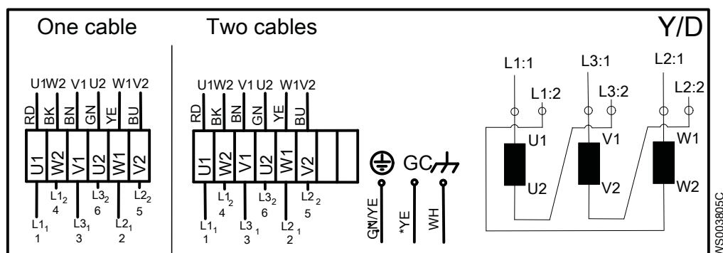
Рис. 10: «Звезда»/«Треугольник»
