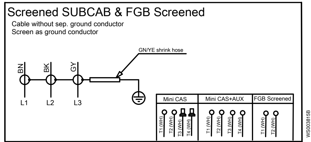
Рис. 14: Экранированный кабель SUBCAB и экранированный кабель FGB
