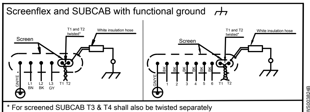
Рис. 15: Кабели Screenflex и SUBCAB с функциональным заземлением
