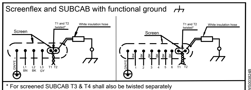
Рис. 15: Кабели Screenflex и SUBCAB с функциональным заземлением
