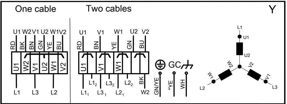
Рис. 8: Соединение “звездой”
