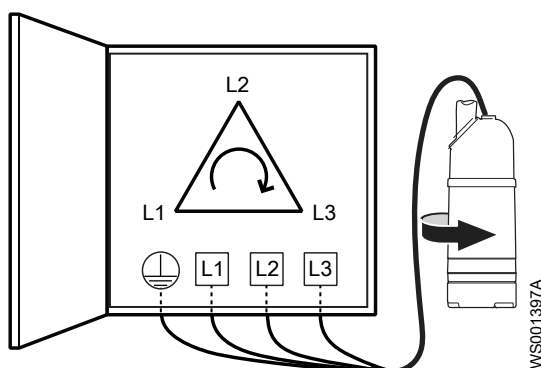
Рис. 3: Включите насос
